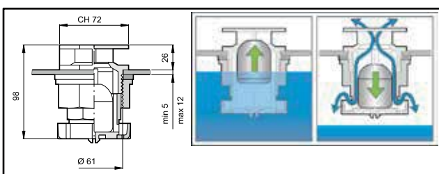
Entlüftungs-Labyrinthventil
