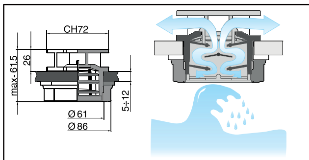
Поплавковый клапан
