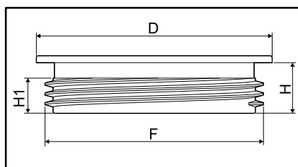
Закрытая крышка
