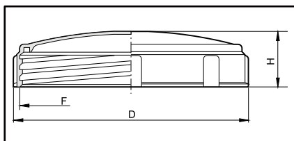
Закрытая крышка
